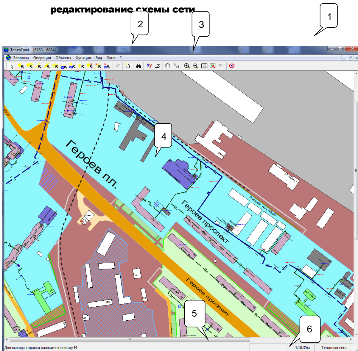
Рисунок 3.2 - Интерфейс ИГС «ТеплоГраф» в режиме Рисование и редактирование схемы сети
