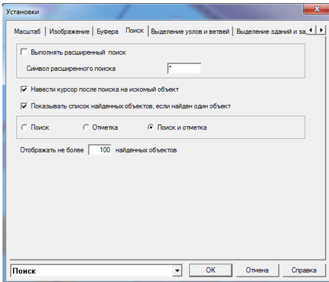
Рисунок 3.79 – Меню Поиск
