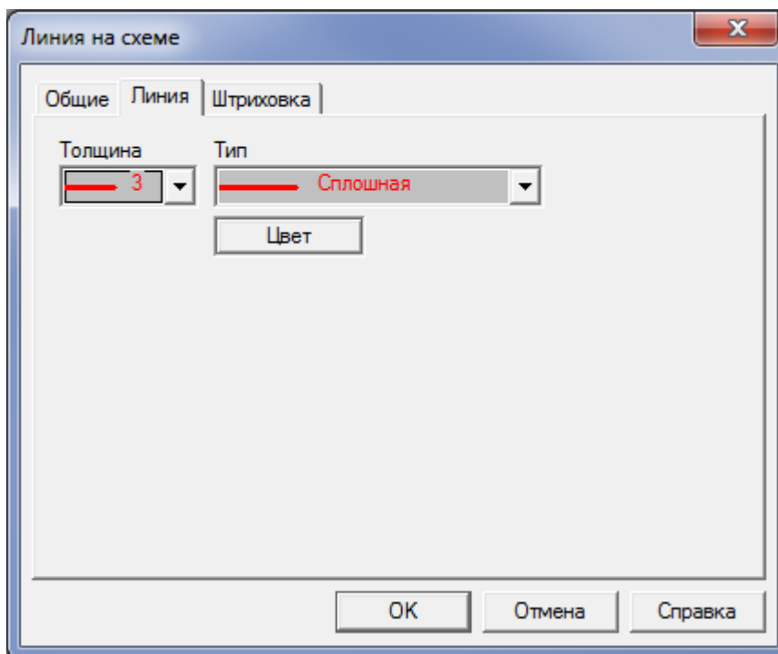
Рисунок 3.156 – Меню Линия
