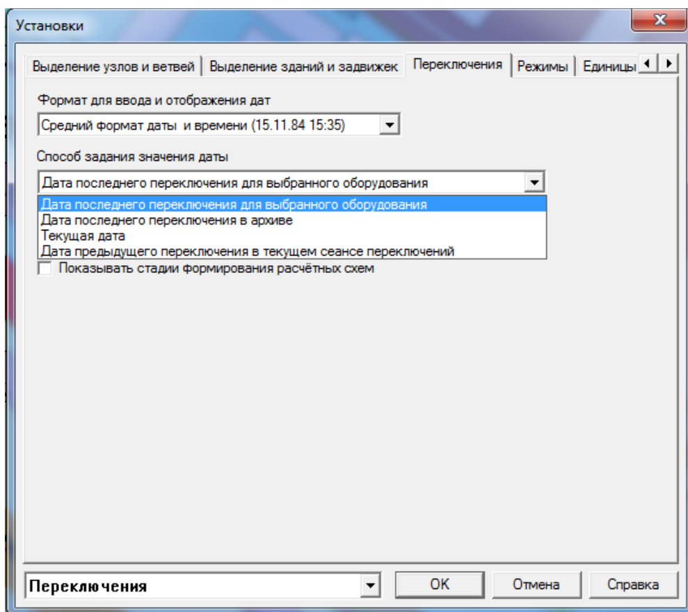
Рисунок 3.129 – Меню Установки
