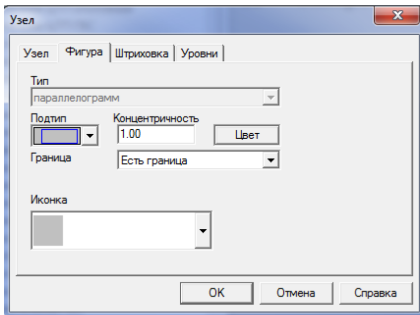
Рисунок 3.138 – Меню Фигура
