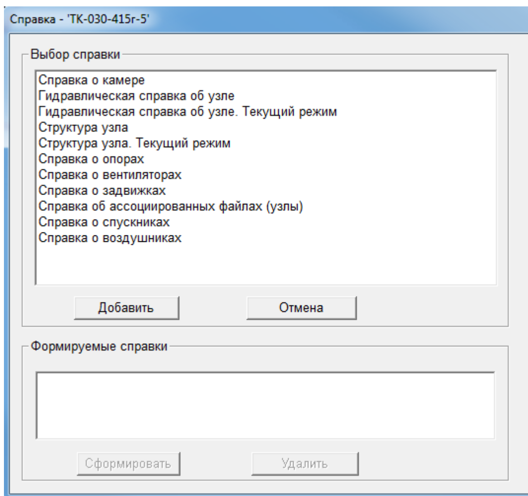
Рисунок 3.98 – Меню Справка
