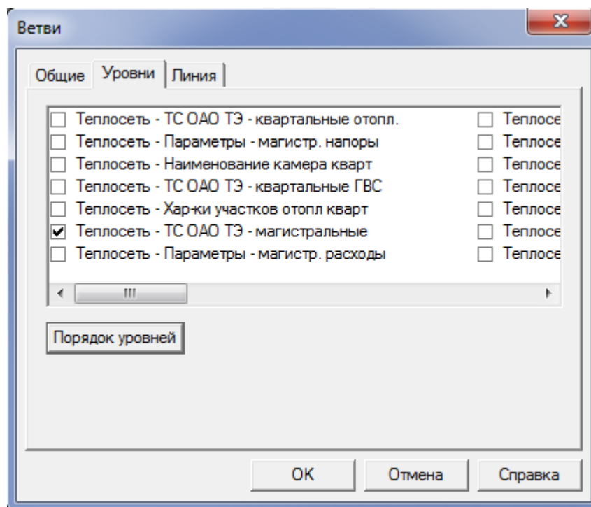
Рисунок 3.144 – Меню Уровни
