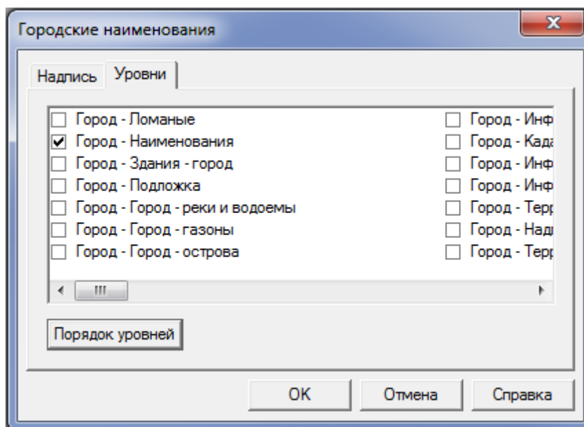
Рисунок 3.153 – Меню Уровни
