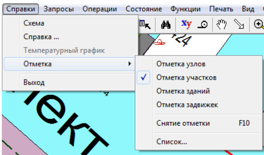
Рисунок 3.108 – Меню Отметка
