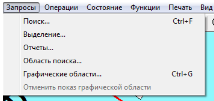
Рисунок 3.110 – Меню Запросы
