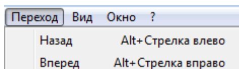
Рисунок 3.103 – Меню Переход
