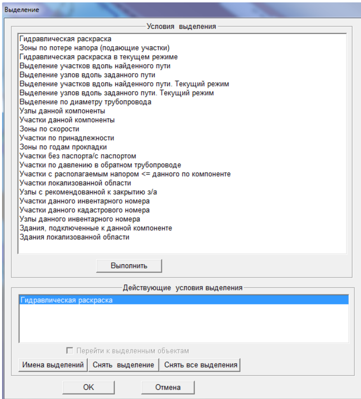
Рисунок 3.9 – Меню Выделение
