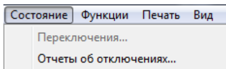
Рисунок 3.115 – Меню Состояние
