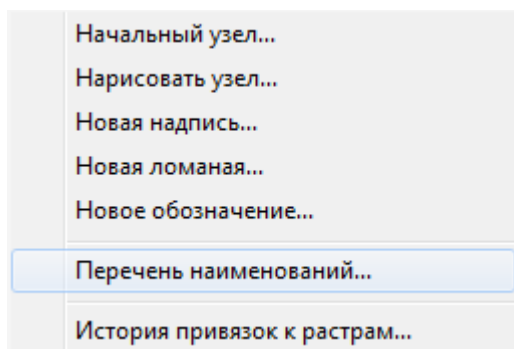
Рисунок 3.52 – Меню Наименования
