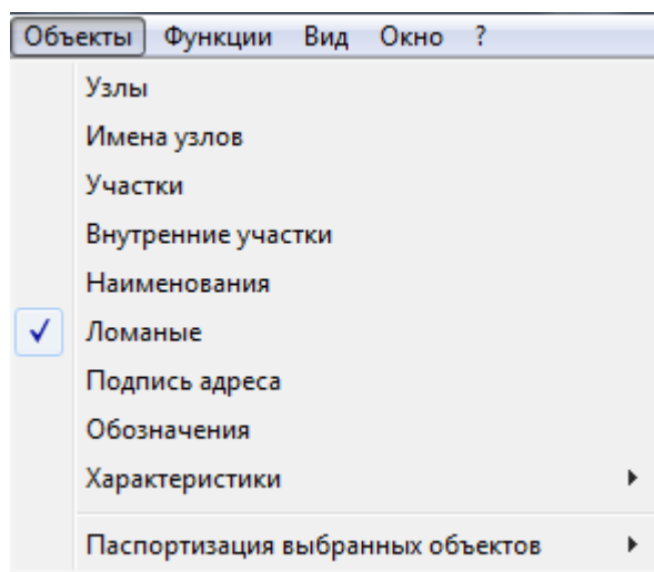
Рисунок 3.26 – Меню Объекты
