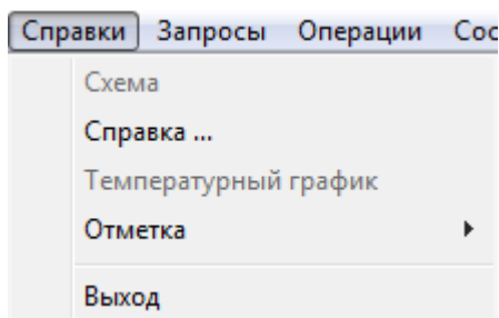
Рисунок 3.96 – Меню Справки
