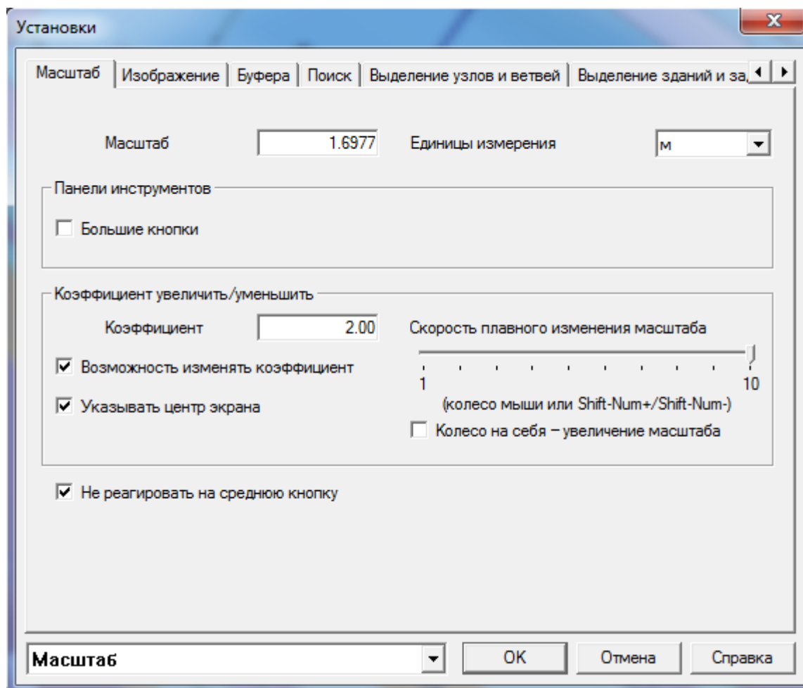
Рисунок 3.77 – Меню Установки
