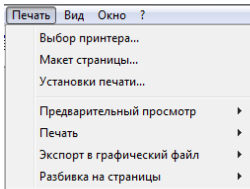
Рисунок 3.125 – Меню Печать
